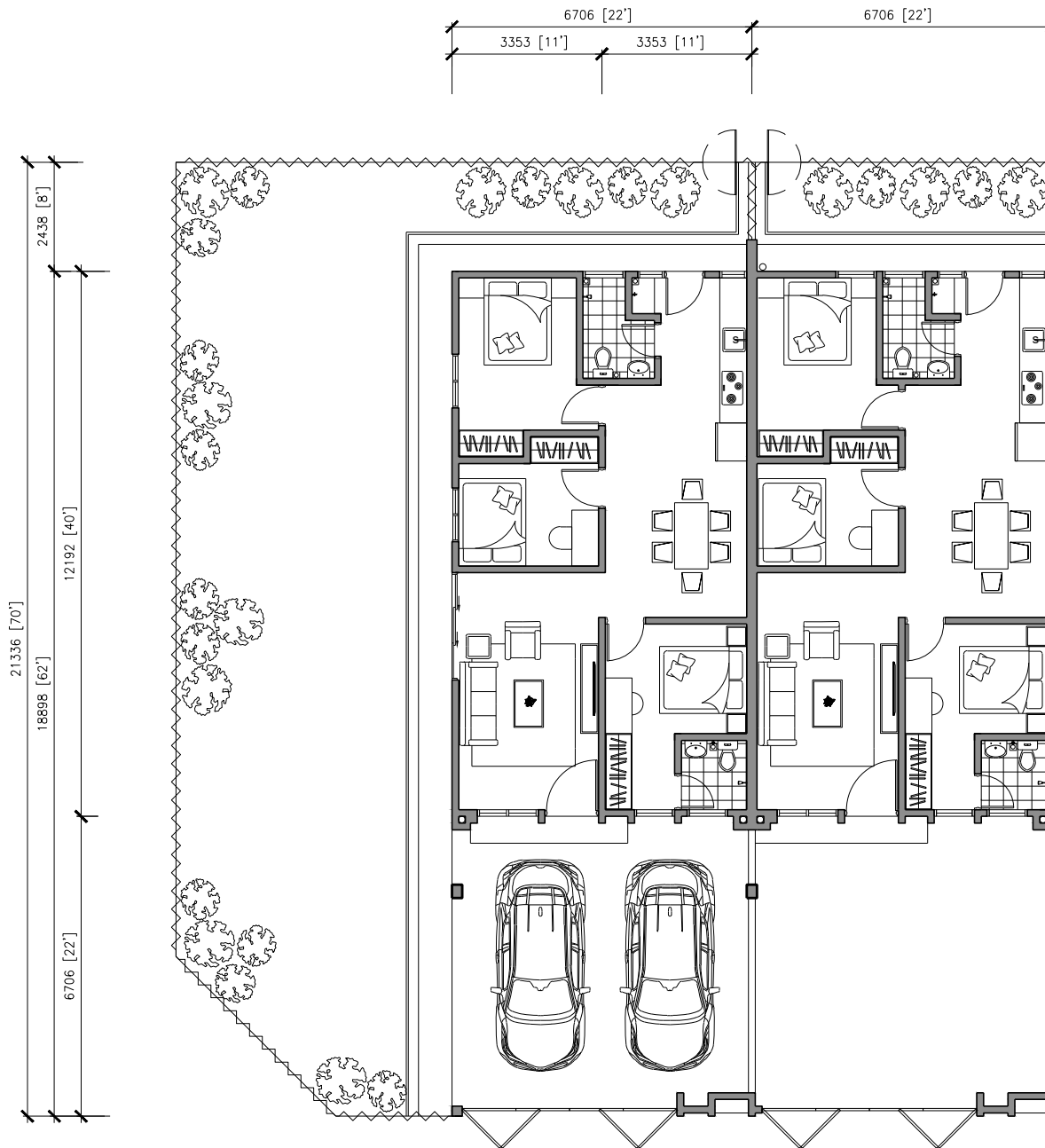
PELAN LANTAI TINGKAT BAWAH (JENIS B)
